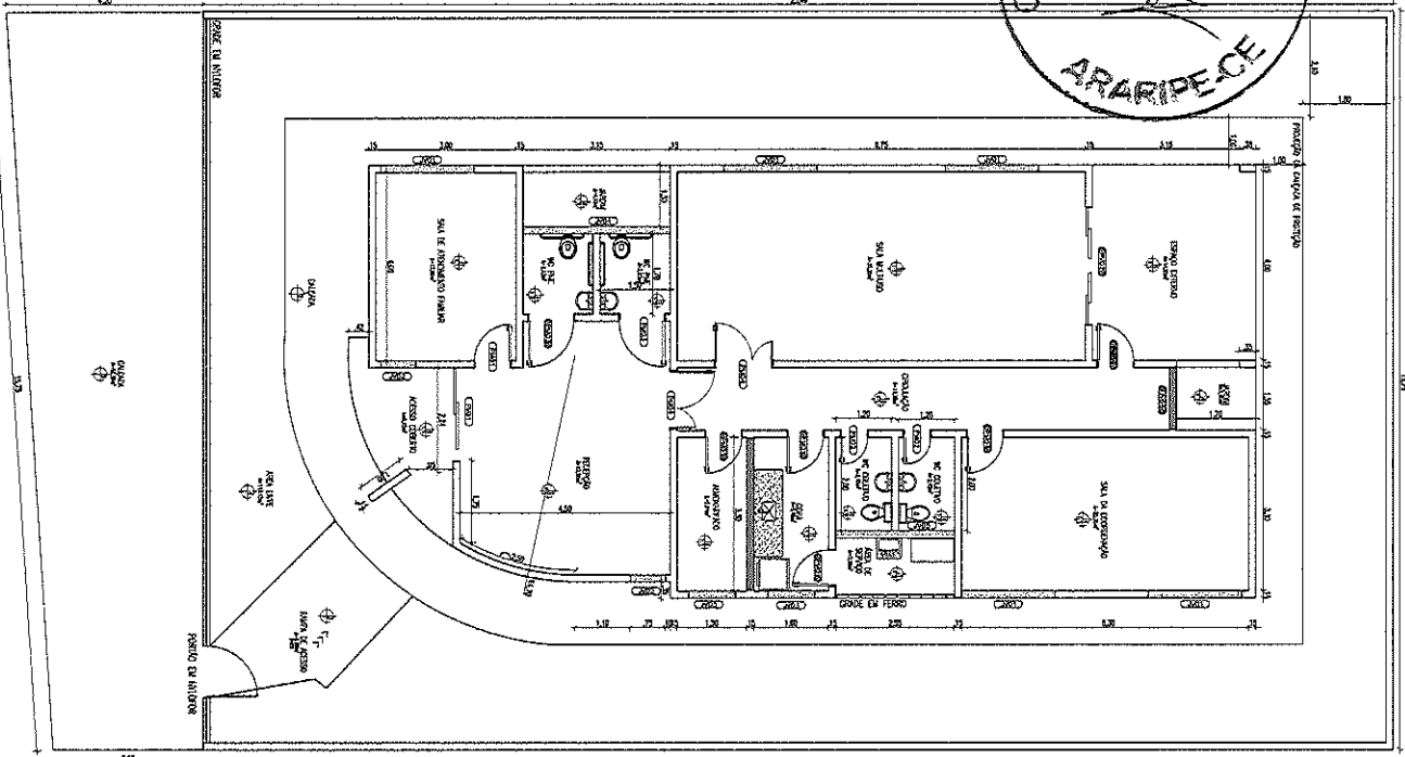
PLANTA BAIXA - INTERVENÇÃO 17/7
