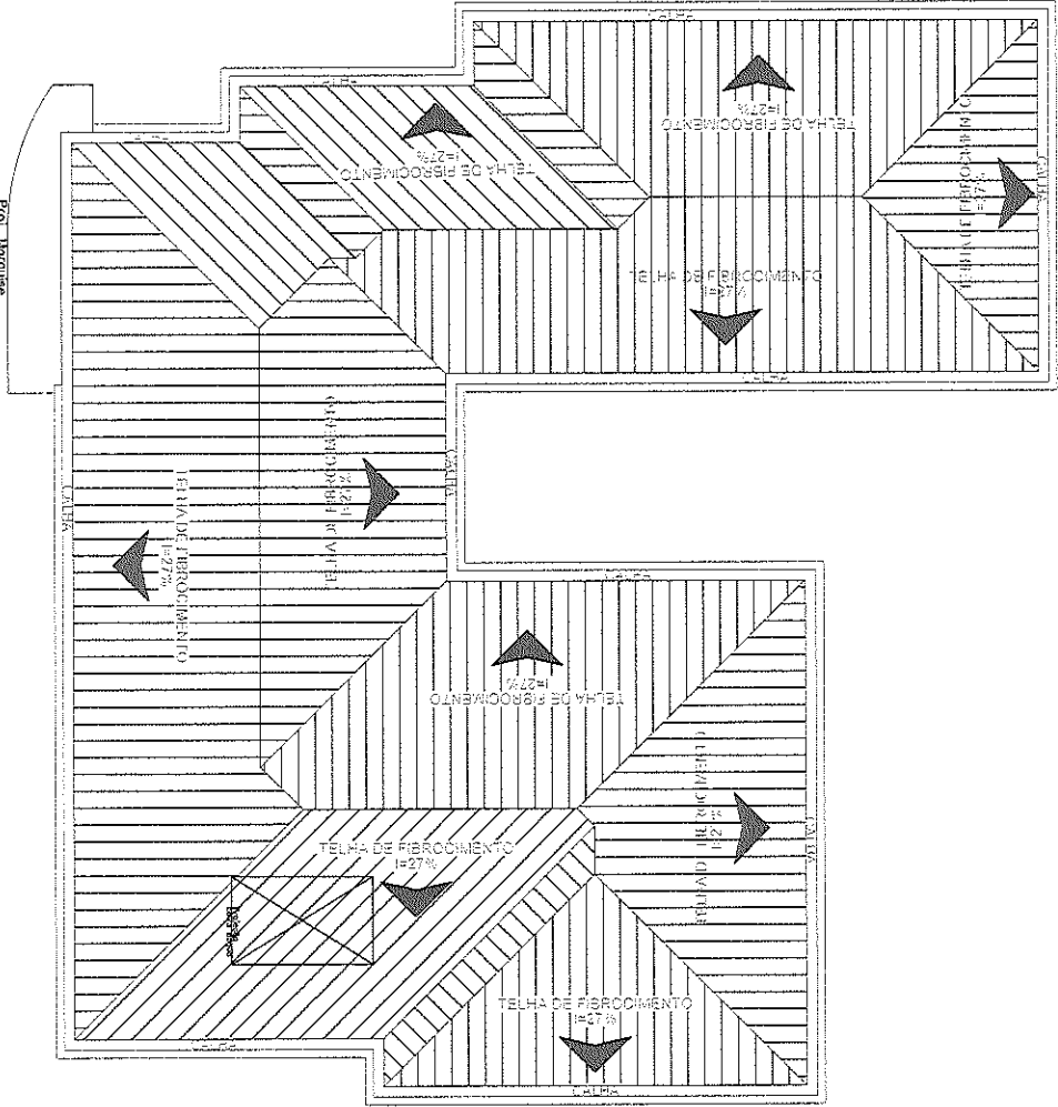
PLANTA DE COBERTA 1/50 ESC.
