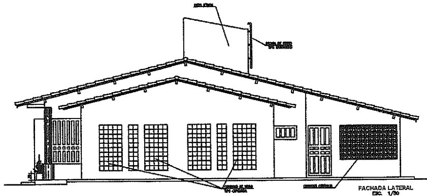
FACHADA LATERAL ESC. 1/50
