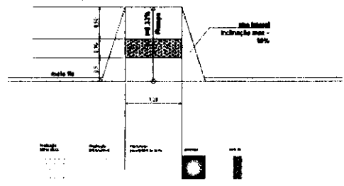
05 PLANTA - RAMPA SEM ESCALA
